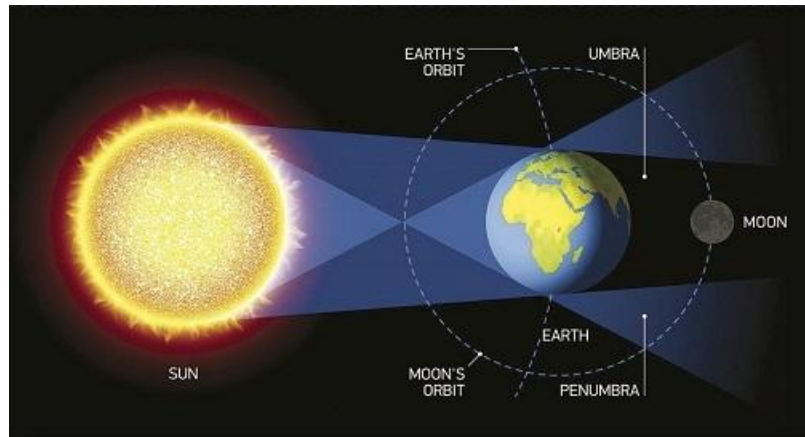
Fig.a) Configurazione dell'Eclissi Totale di Luna
